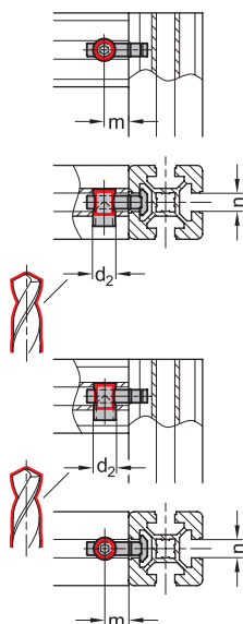
Montaje/mecanizado de perfiles
