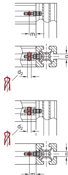
Montaje/mecanizado de perfiles
